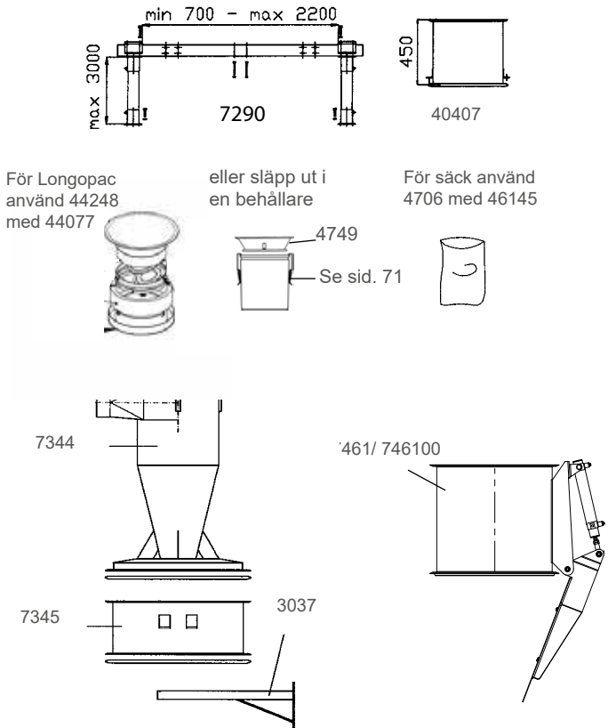
F 8000 Stationary levereras med cyklon, magasin och 2 konsoler för väggmontage
