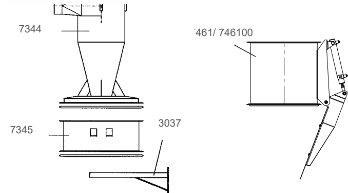
F 8000 Stationary levereras med cyklon, magasin och 2 konsoler för väggmontage
