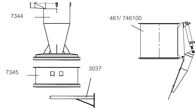
F 8000 Staionary levereras med cyklon, magasin och 2 konsoler för väggmontage
