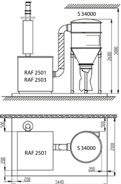
RAF 2501 / 2503, S 34000
