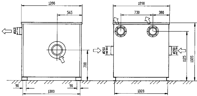
Dimensions RAF 2502
