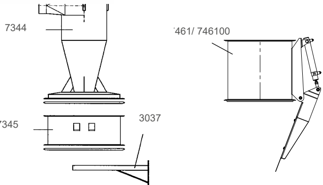
F 8000 Stationary levereras med cyklon, magasin och 2 konsoler för väggmontage
