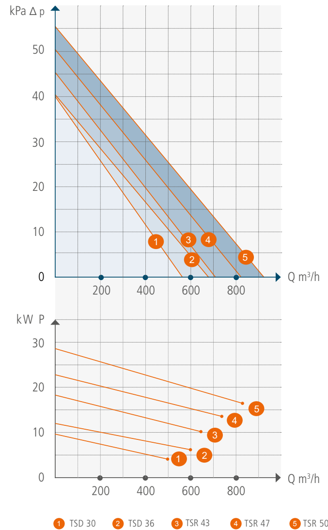
Turbopumparna TSD/TSR
