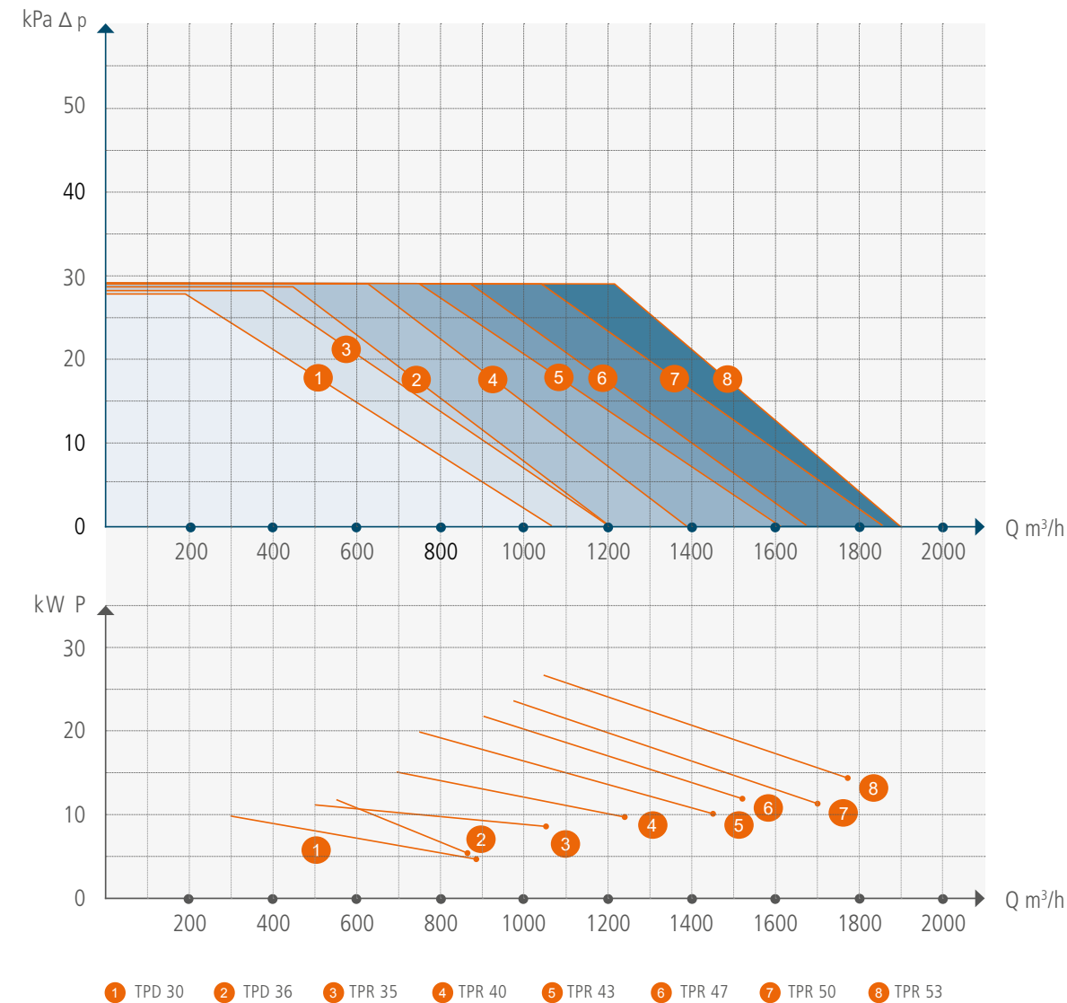
Turbopumparna TPD/TPR
