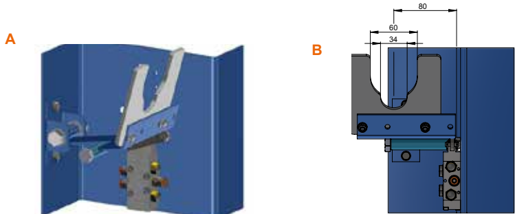
A Hållare för handhållna verktyg B Fjäderbelastad 5/2-ventil (styr skjutspjället i utsugningssystemet)
