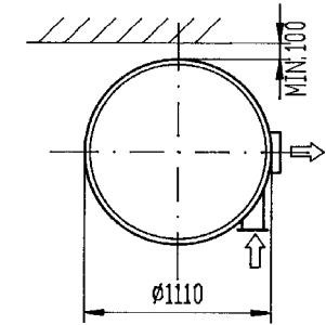
F 30000 med art.nr 4706 Utmatningskona och 4612 Modulring
