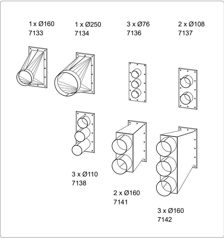
Inloppsmoduler för F 20000 och F 30000 (art.nr)
