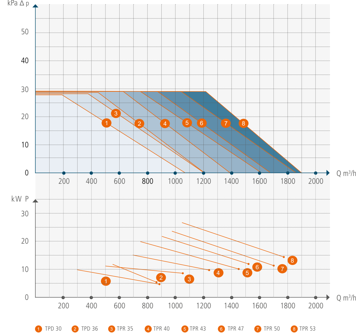
Turbopumps TPD/TPR
