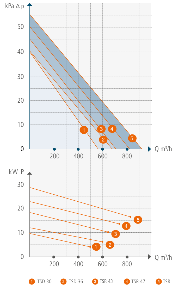
Turbopumps TSD/TSR
