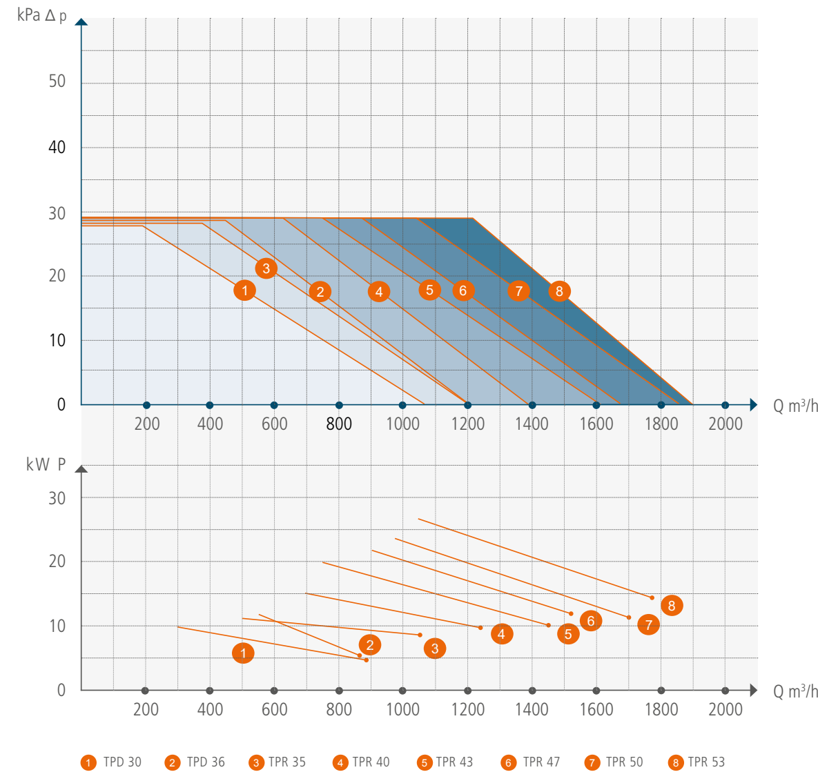
Turbopumparna TPD/TPR
