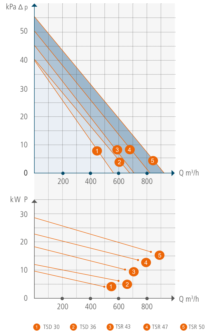
Turbopumps TSD/TSR
