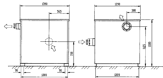
Dimensions RAF 2501 / RAF 2503
