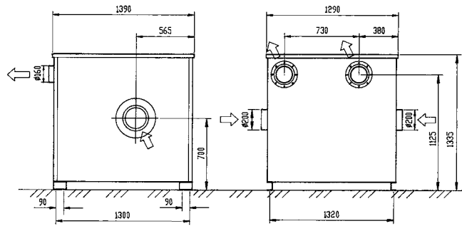
Dimensions RAF 2502
